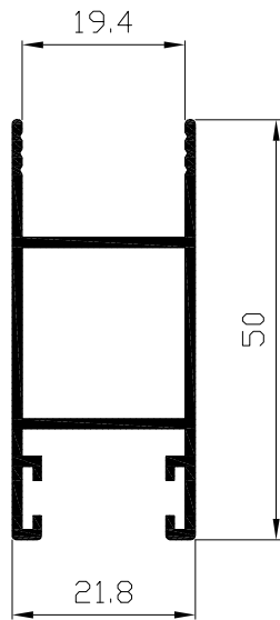
Hoja lateral 50 vidrio c.cámara Ref: 2533
