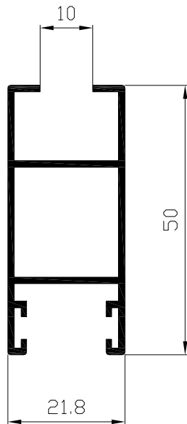
Hoja lateral 50 vidrio simple Ref: 2126
