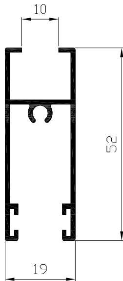
Hoja ruedas vidrio simple Ref: 2104
