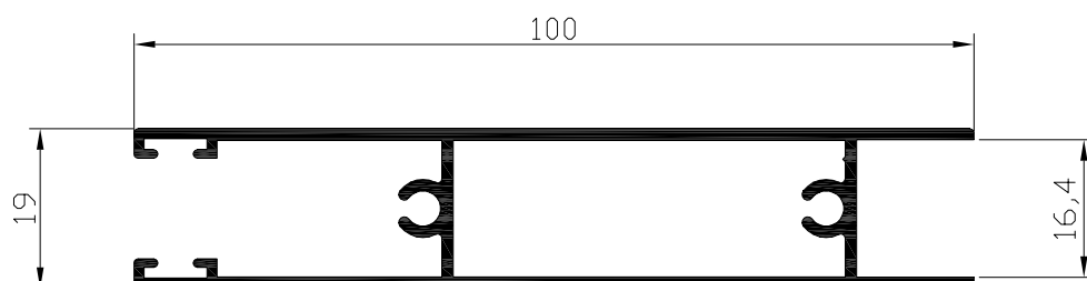
Zócalo vidrio c.cámara Ref: 2117
