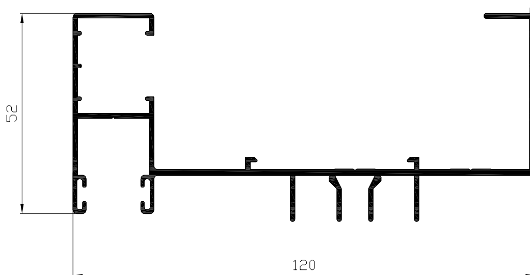
Marco lateral izquierdo c. guia Ref: 2143 (INTEGRAL)
