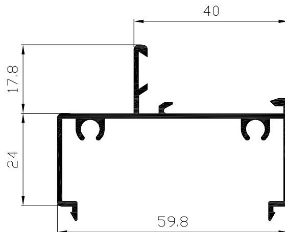
Marco fijo con clip Ref: 2111
