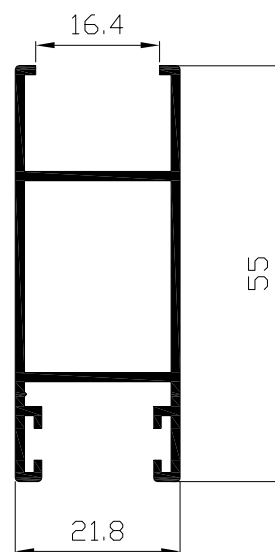
Hoja lateral 55 vidrio c.cámara Ref: 2116
