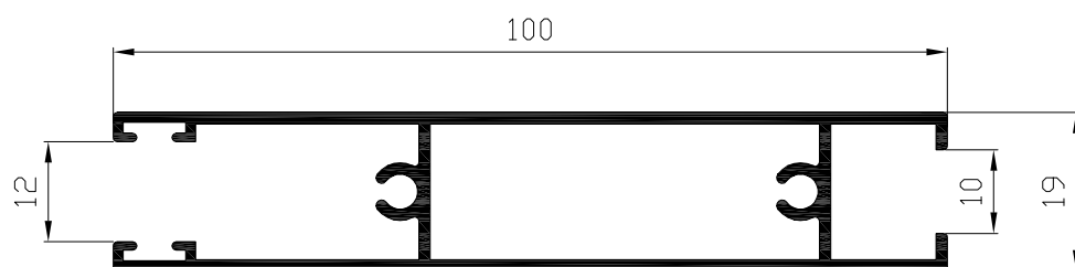
Zócalo vidrio simple Ref: 2107
