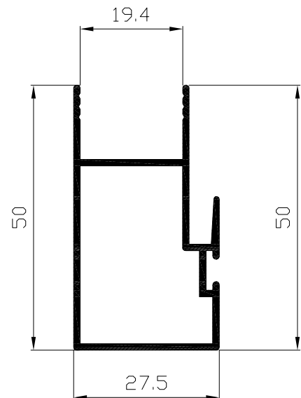
Hoja central vidrio c.cámara Ref: 2532
