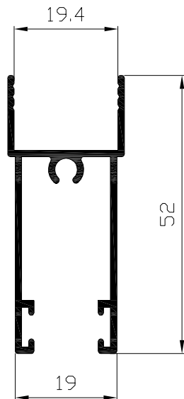
Hoja ruedas vidrio c.cámara Ref: 2531
