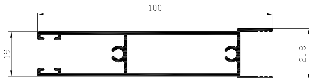
Zócalo vidrio c.cámara Ref: 2657
