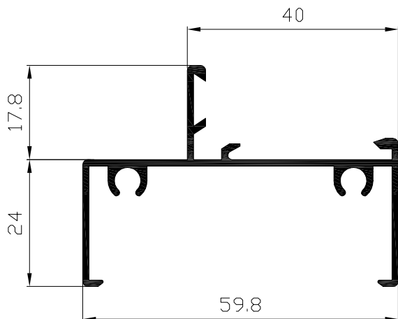
Marco fijo sin clip Ref: 2112
