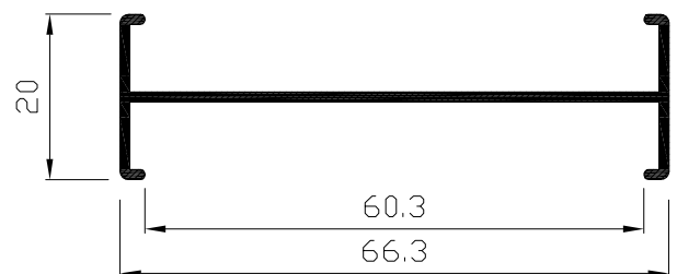
Unión de marcos Ref: 2211
