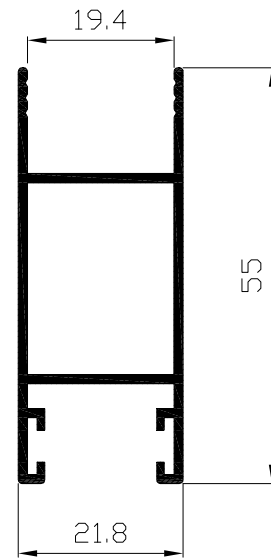
Hoja lateral 55 vidrio c.cámara Ref: 2534
