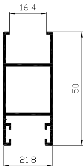
Hoja lateral 50 vidrio c.cámara Ref: 2136
