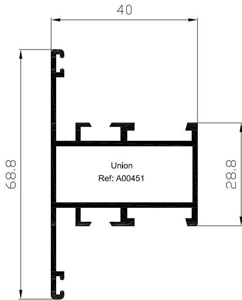
Travesaño ventana Ref: 4008
