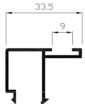
Junquillo zócalo Ref: 4107
