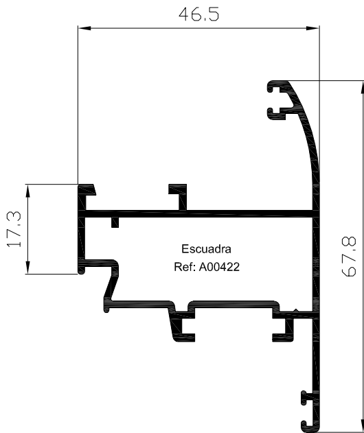
Hoja apert.ext ventana 40 Ref: 4014
