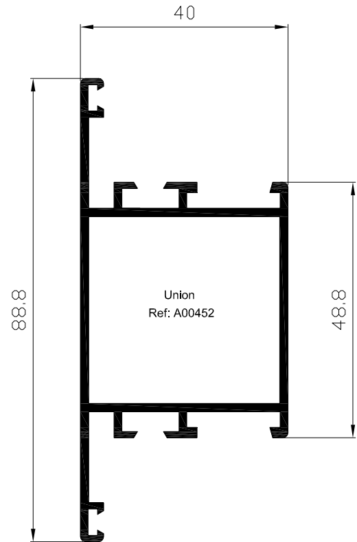
Travesaño puerta Ref: 4018
