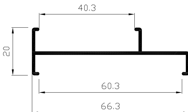
Unión bandera SELECT-60 Ref: 2212
