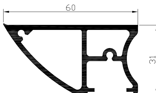
Refuerzo-tirador hoja Ref: 9113
