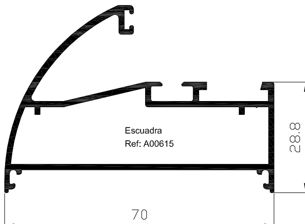
Marco fijo 70 mm Ref: 7111
