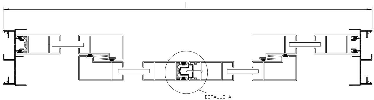
DETALLE A
