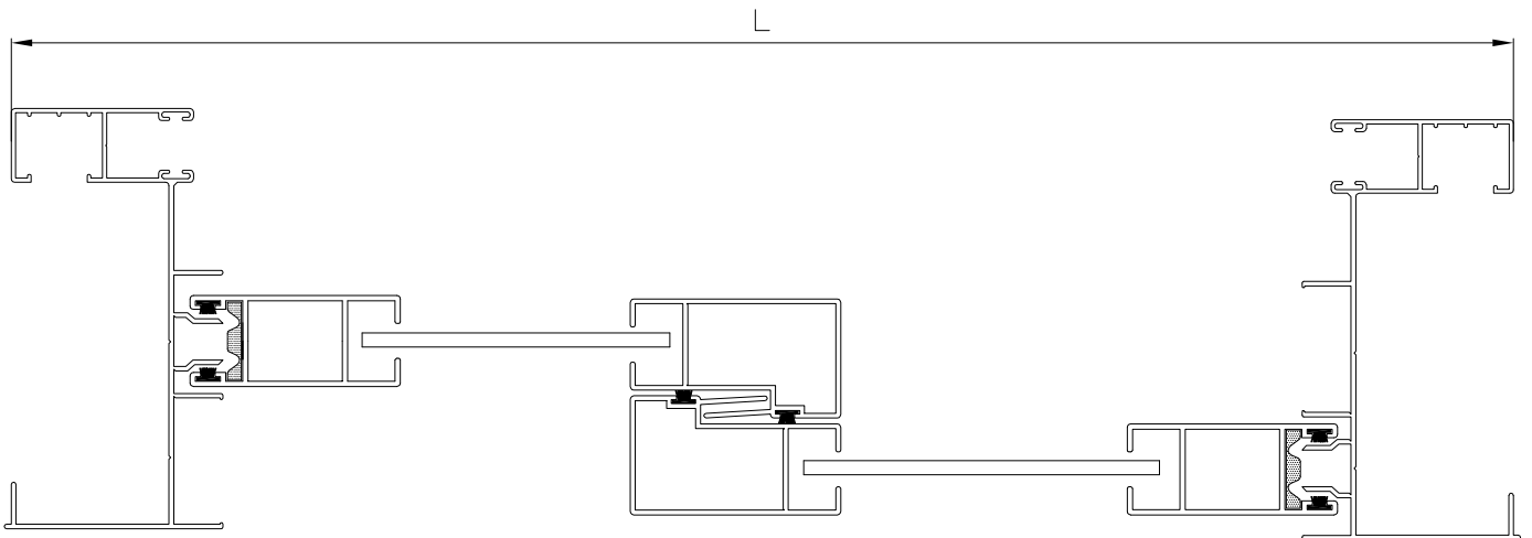
SECCION B-B'
