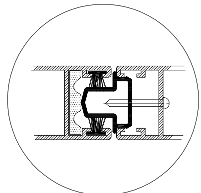
DETALLE A
