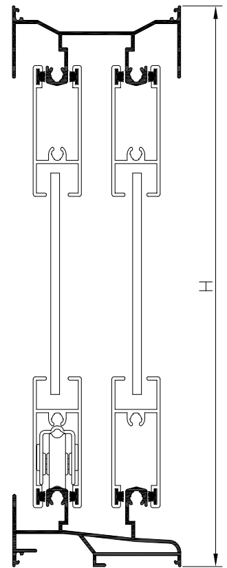
SECCION A-A'
