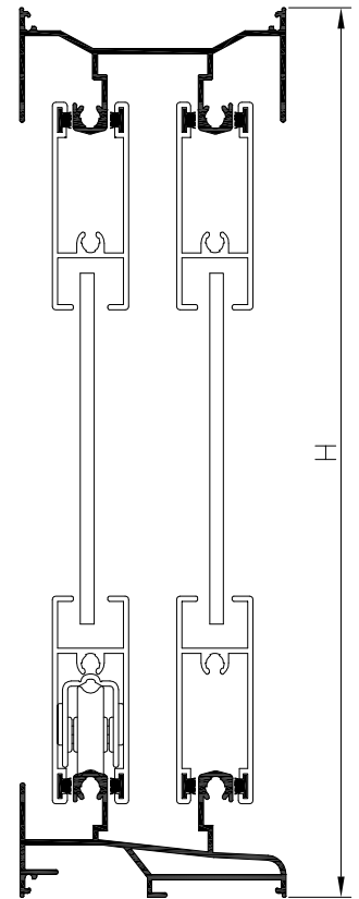
SECCION A-A'
