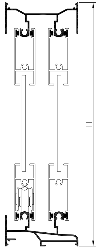
SECCION A-A'
