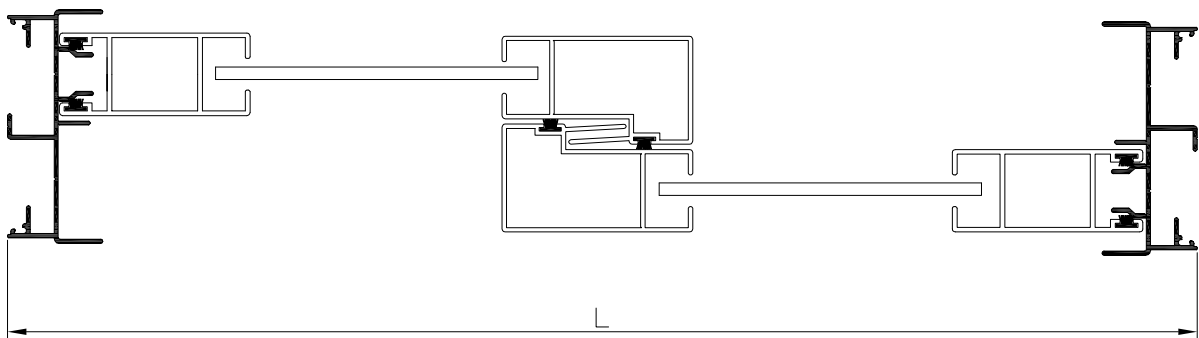
SECCION B-B'
