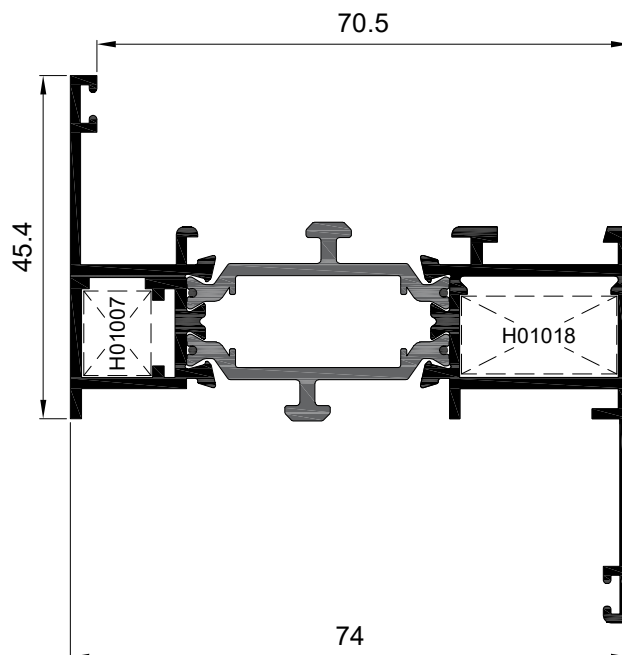
Marco ventana con solape Ref: 7621
