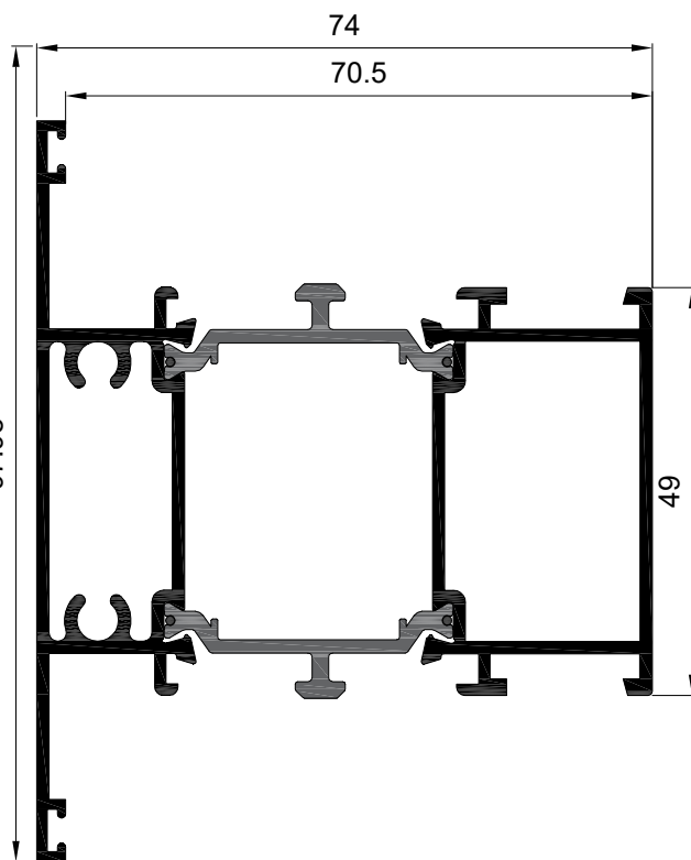
Travesaño zocalo Ref: 7607
