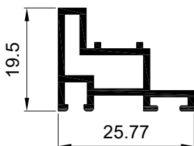
Perfil inferior puerta con pisadera Ref: 5529
