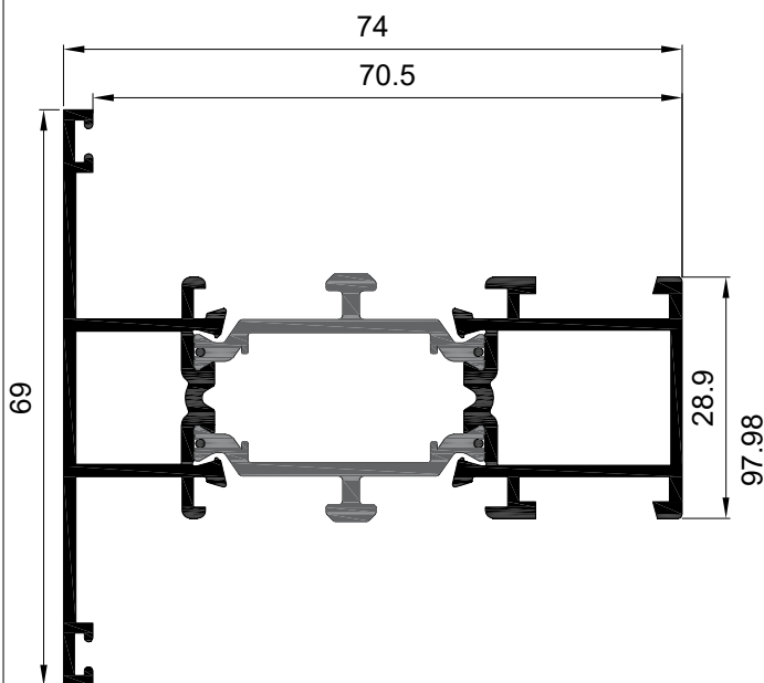
Travesaño ventana Ref: 7608
