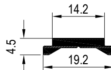
Pletina Falleba Aluminio Ref.- 4110
