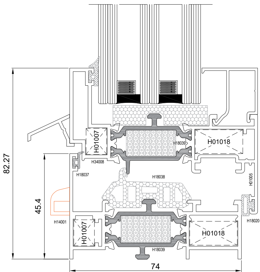
SECCION VERTICAL (A-A*)
