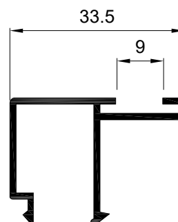
Junquillo zócalo Ref: 4107
