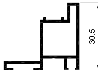
Perfil inferior puerta sin pisadera Ref: 5519
