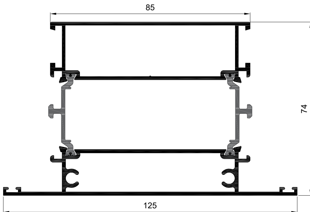
Travesaño zocalo Ref: 7607
