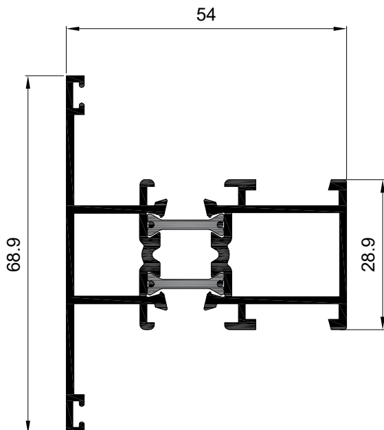
Travesaño ventana Ref: 5508
