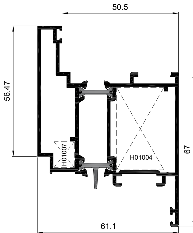
Hoja Puerta Ap.Interior Ref: 5505
