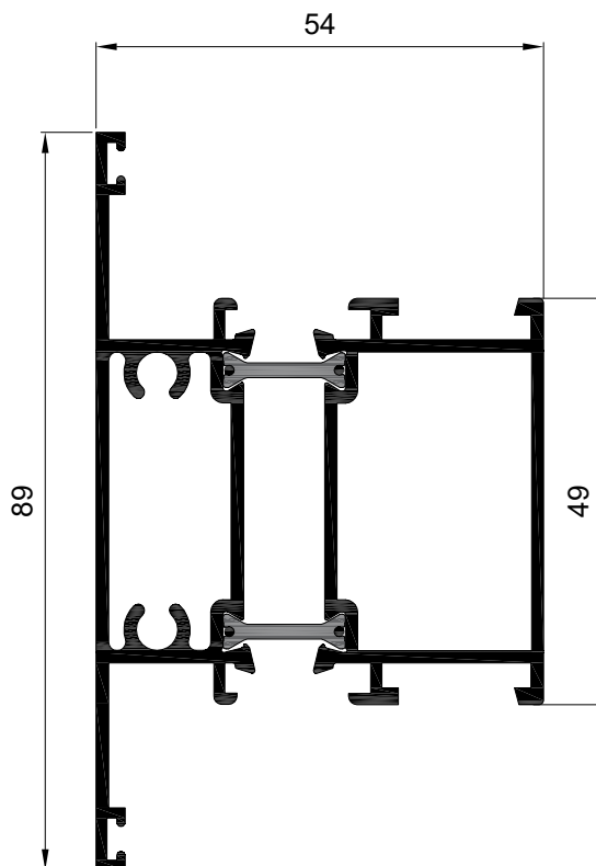
Travesaño puerta Ref: 5518
