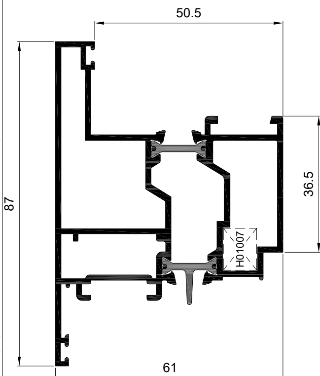
Hoja Puerta Ap.Exterior Ref: 5515
