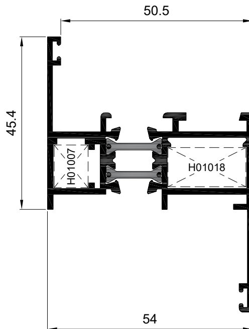
Marco ventana con solape
