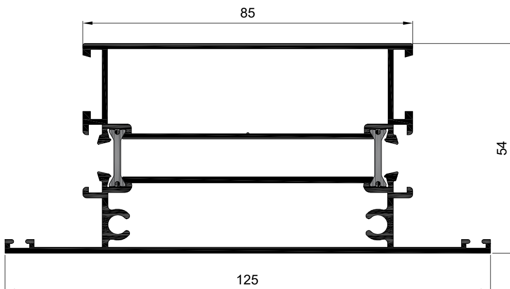
Travesaño zocalo Ref: 5507
