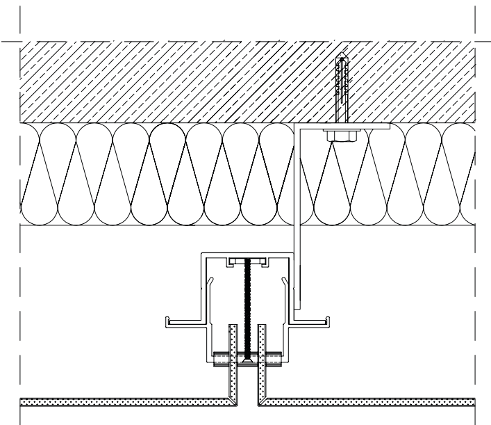
HORIZONTAL A-A'
