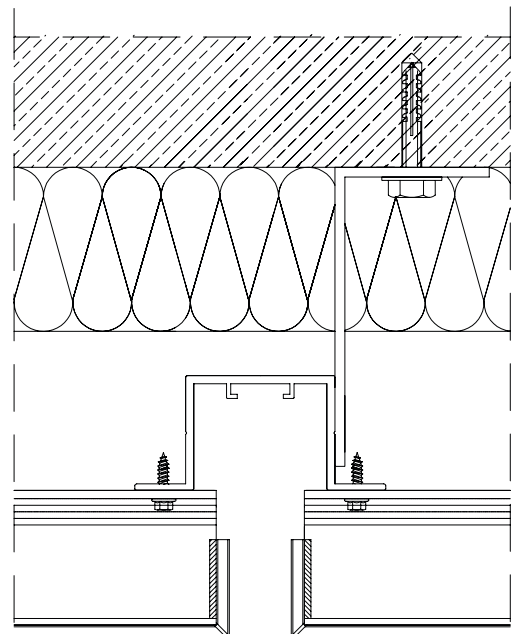
HORIZONTAL B-B'
