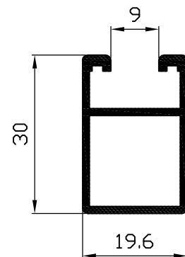
Hoja de una salida Ref: 1008
