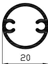
Redondo autorroscante Ref: 1024
