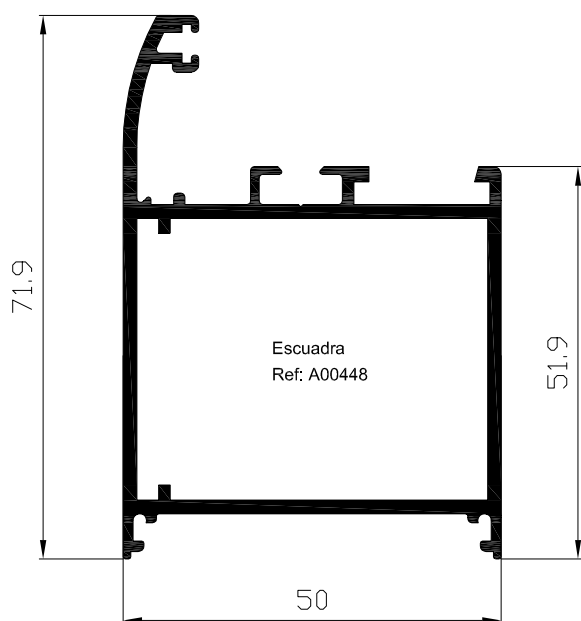
Marco fijo Ref: 4621
