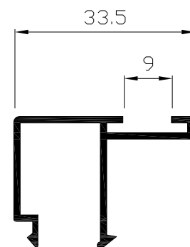
Junquillo zócalo Ref: 4107
