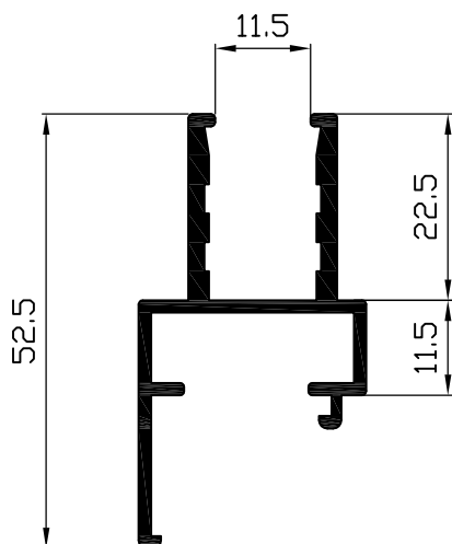
Portavidrios atornillado Ref: 1038
