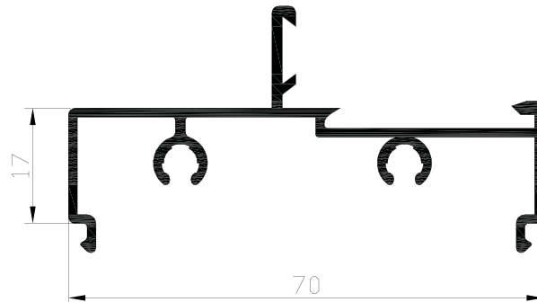
Marco fijo c.clip Ref: 7N11
