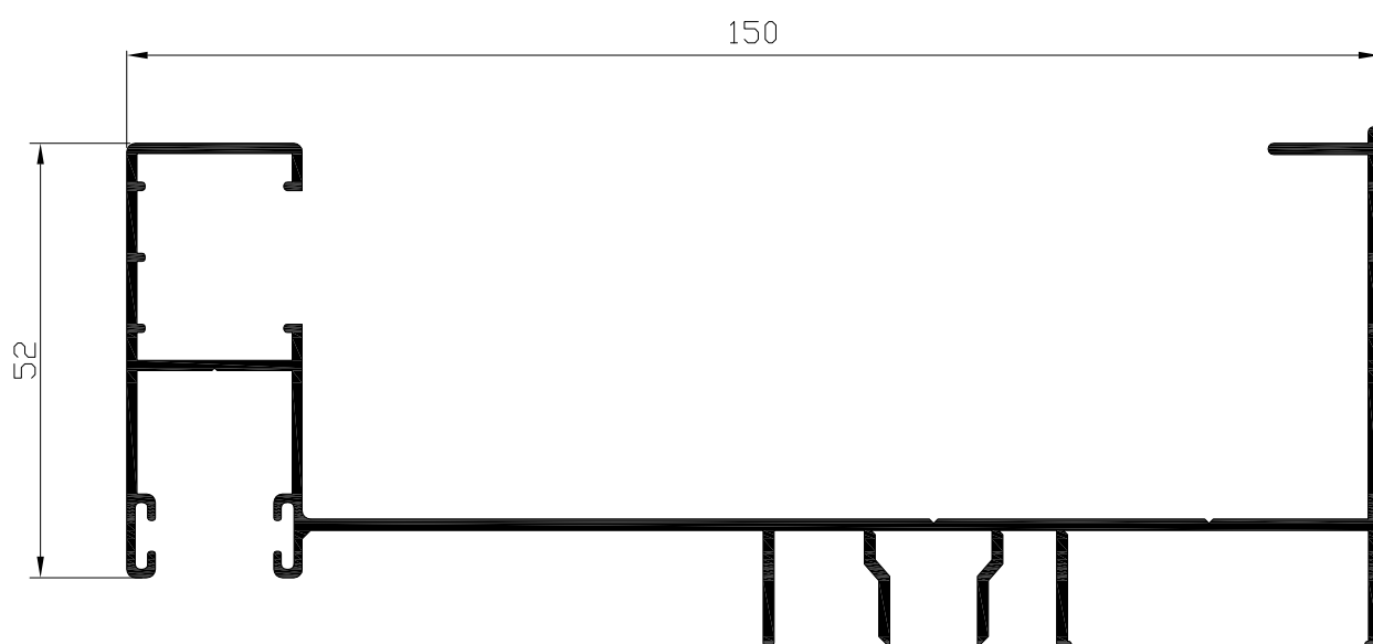
Marco lateral izquierdo con guia Ref: 7054 (INTEGRAL)
