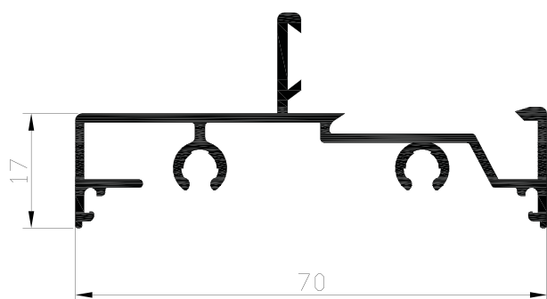
Marco fijo s.clip Ref: 7N12
