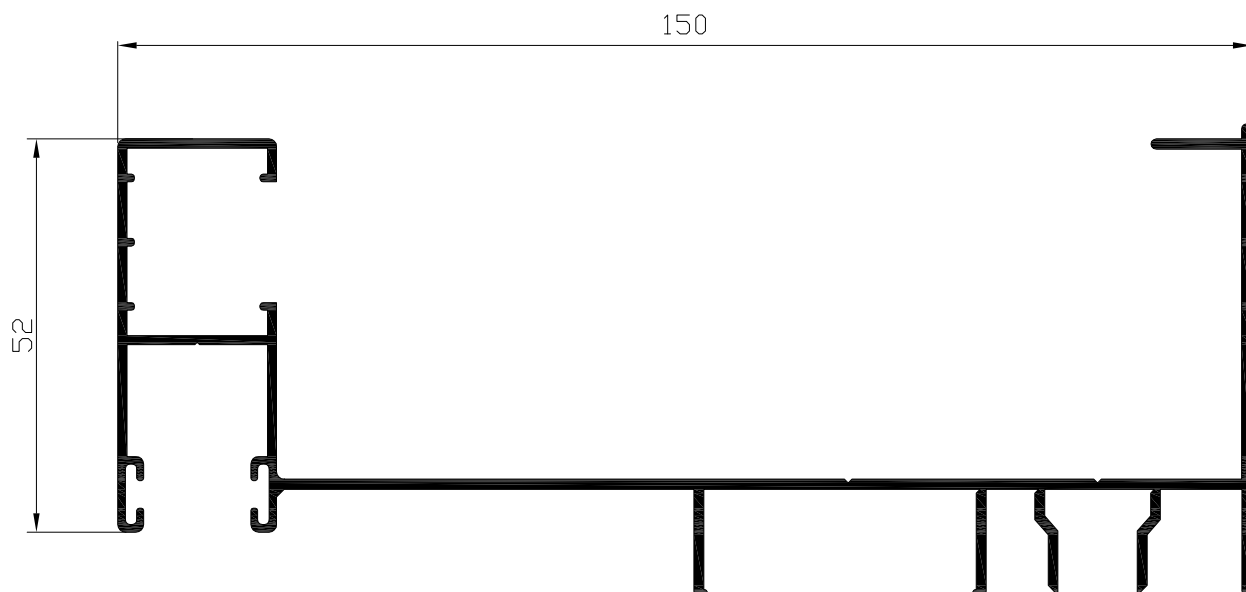
Marco lateral derecho con guia Ref: 7044 (INTEGRAL)
