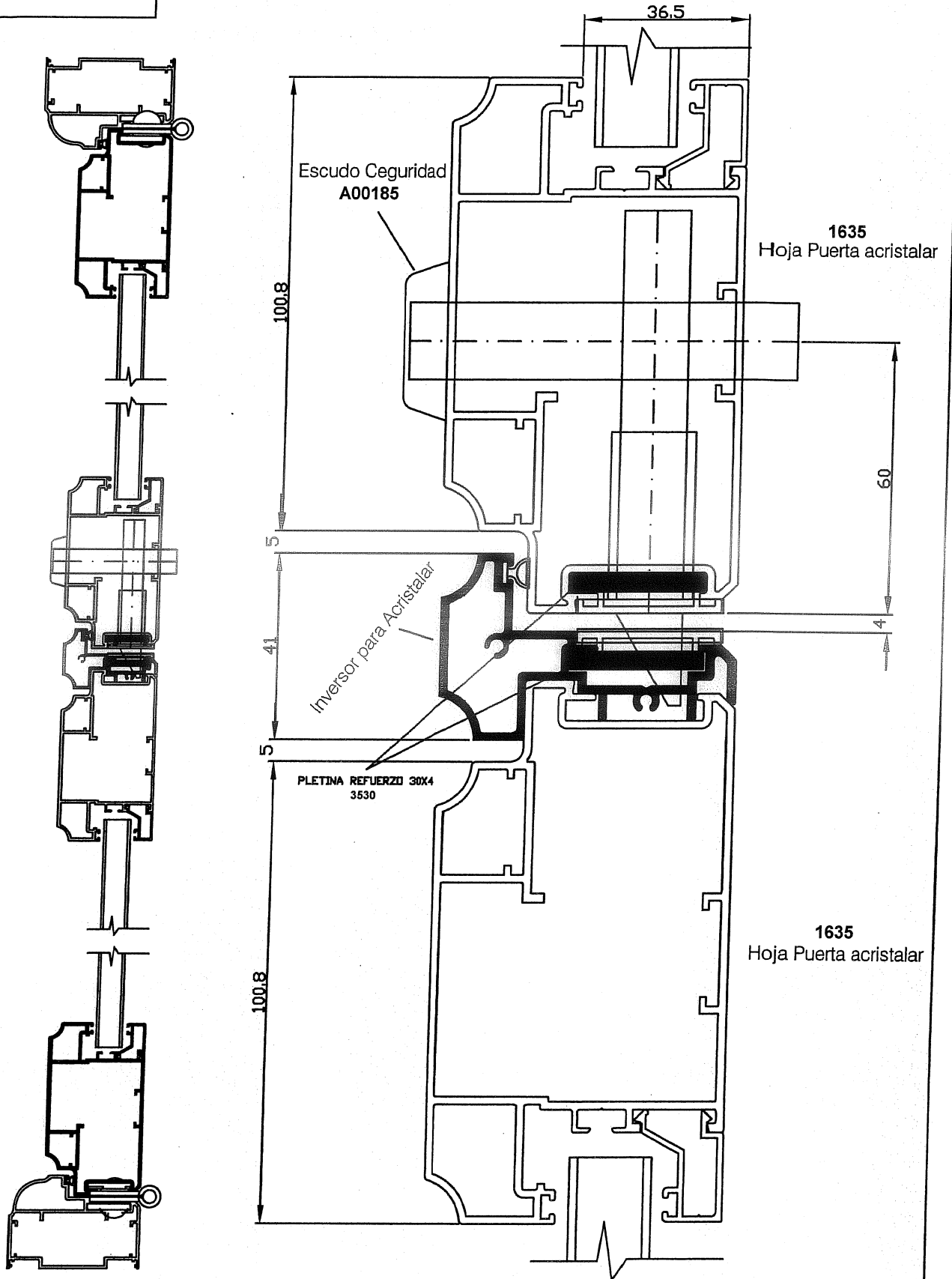
SECCION HORIZONTAL 2 HOJAS
