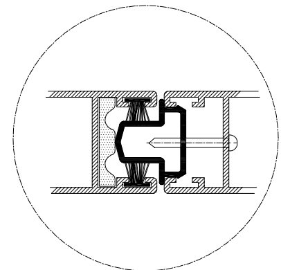
DETALLE A
