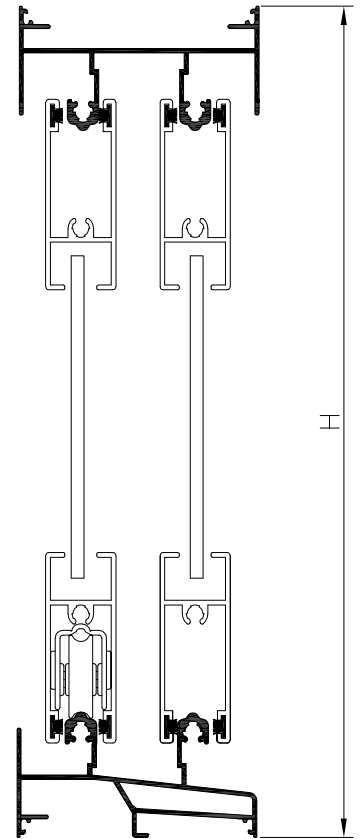
SECCION A-A'
