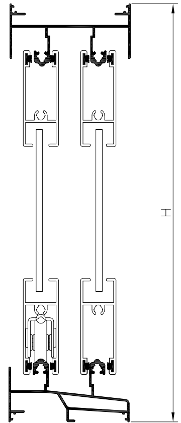
SECCION A-A'
