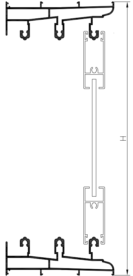
SECCION A-A'
