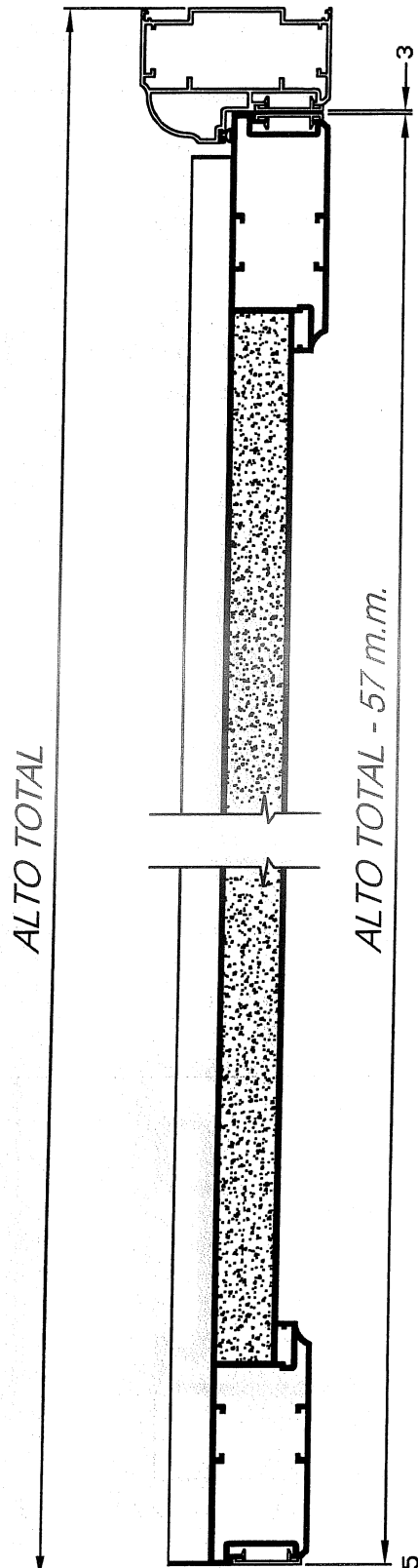
SECCION VERTICAL HOJA CON DUELAS
