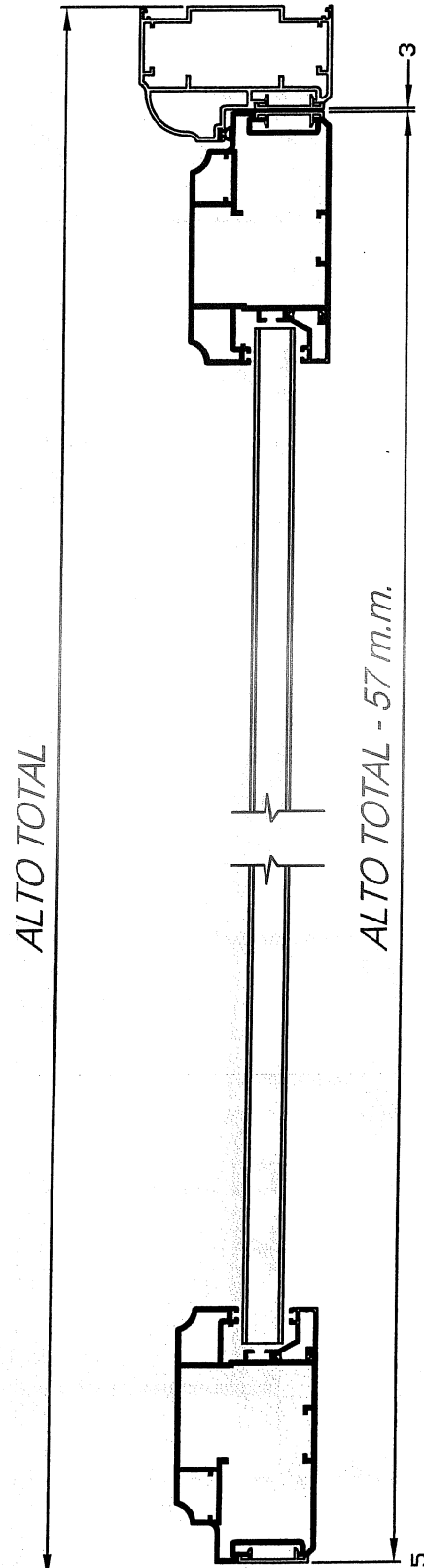
SECCION VERTICAL HOJA DE ACRISTALAR
