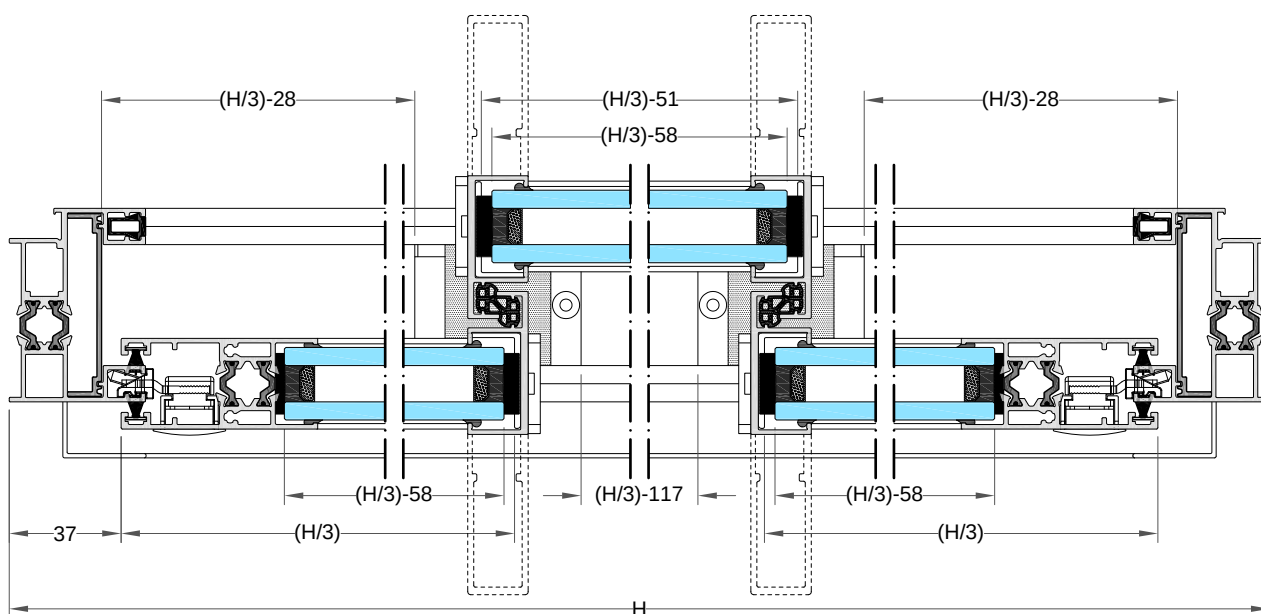
Sección horizontal
