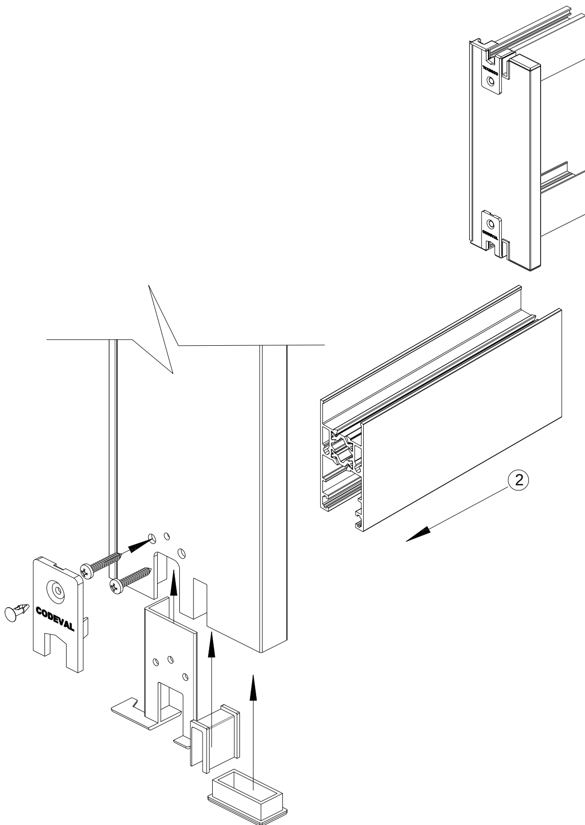
Tapón hoja Ref.: H34056
