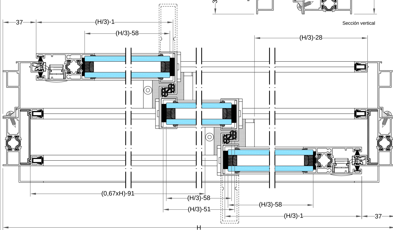
Sección horizontal
