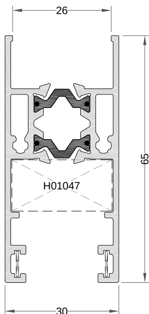
Hoja hueco 26 Ref.: 8414
