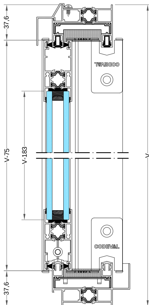
Sección vertical
