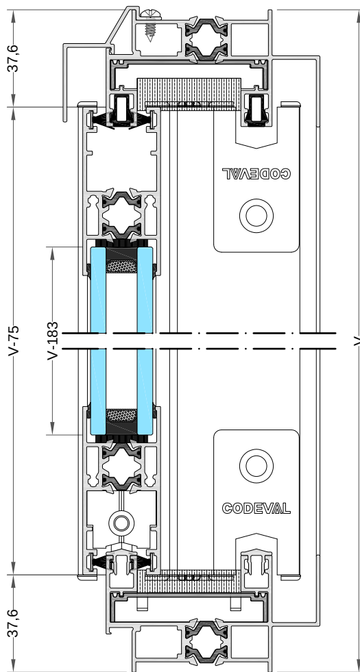
Sección vertical
