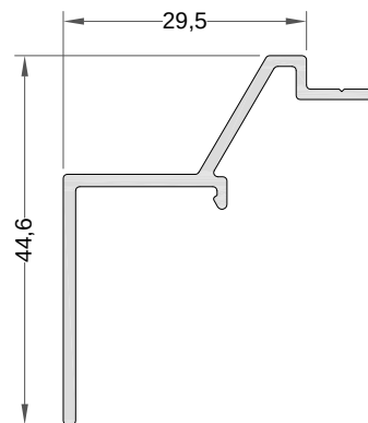
Vierteaguas exterior Ref.:8419
