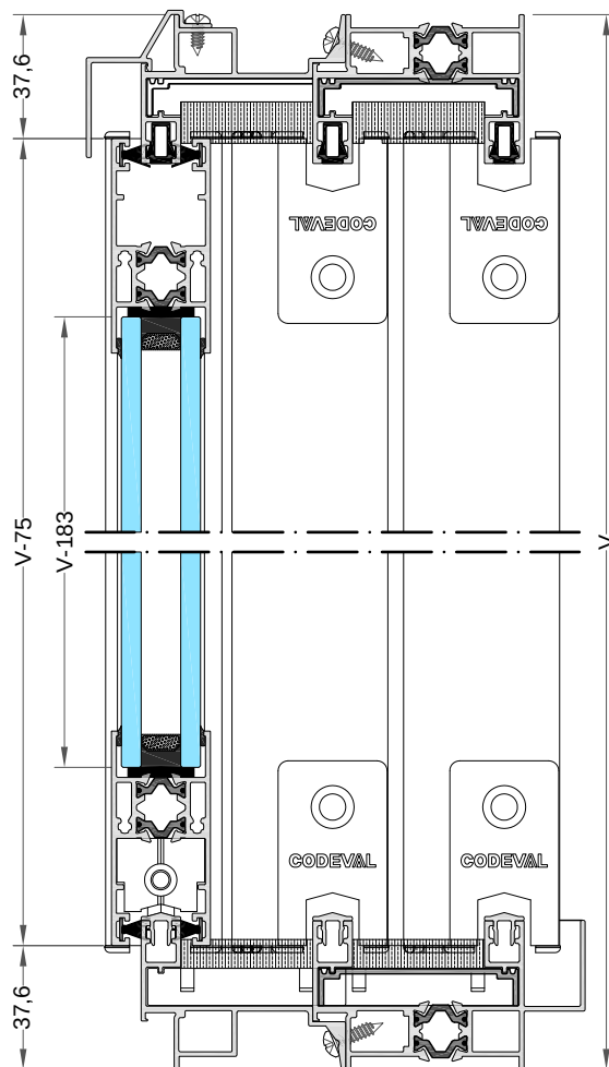
Sección vertical
