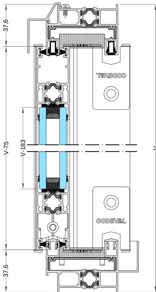
Sección vertical
