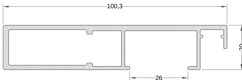
Perfil tirador cruce Ref.: 8405
