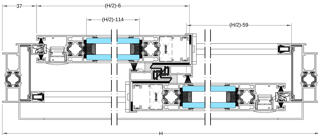
Sección horizontal
