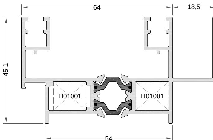
Marco con vierteaguas Ref.: 8402
