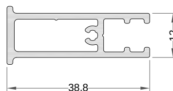
Unión 4 hojas Ref.: 8410
