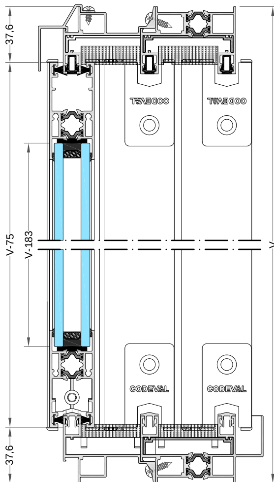
Sección vertical
