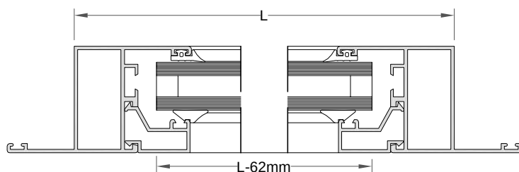
Seccion Horizontal
