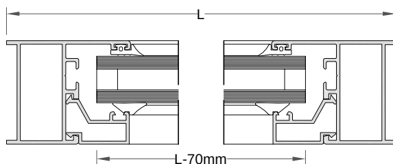
Seccion Horizontal
