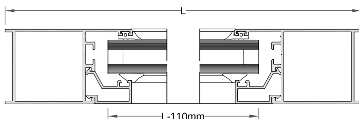
Seccion Horizontal
