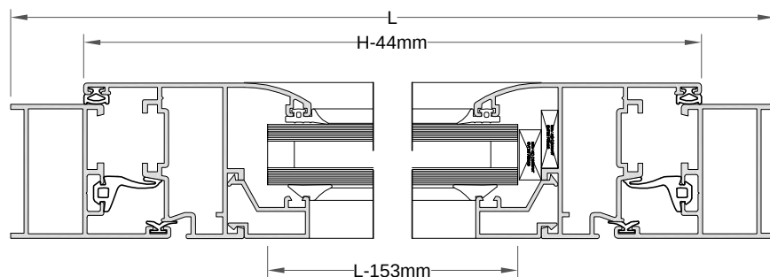
Seccion Vertical
