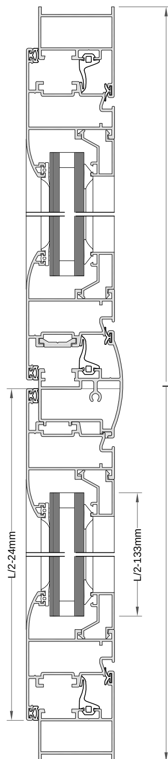
Seccion Horizontal
