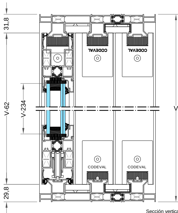
Sección vertical
