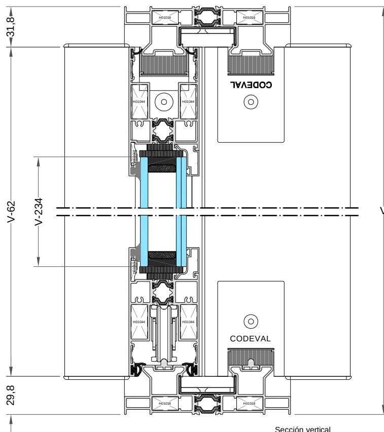
Sección vertical
