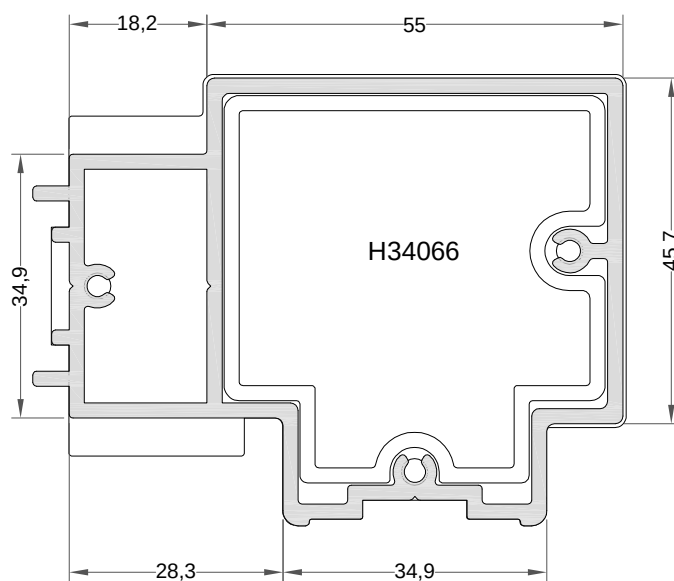
Cantonera móvil Ref.: 7921
