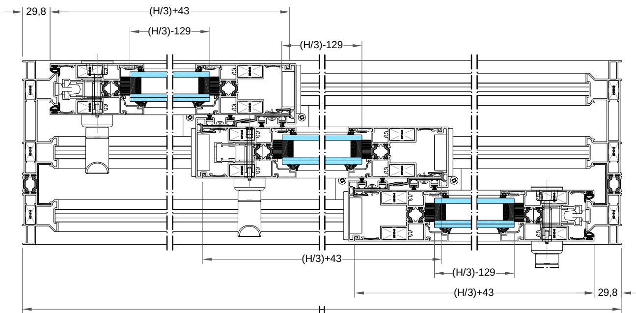
Sección horizontal
