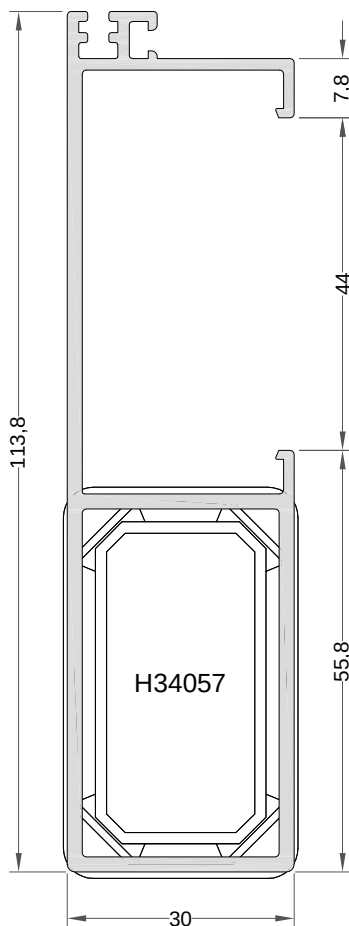
Hoja minimalista reforzada Ref.: 7915
