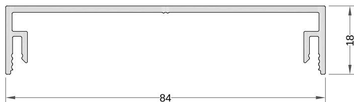
Tapa canal troquelada Ref.: 6703T
