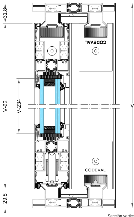
Sección vertical
