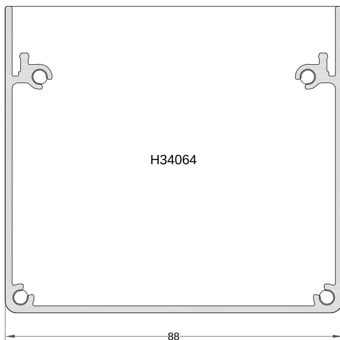
Canal de drenaje Ref.: 7911
