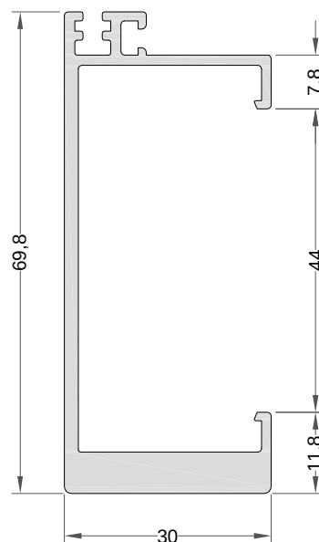
Hoja minimalista Ref.: 7925
