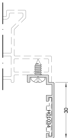
Solape resalte 30 Ref.: 9430
