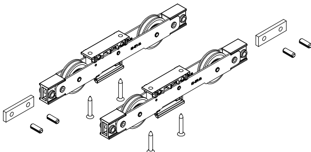
Kit carros intermedios (400 Kg/Hoja) Ref.: H20002
