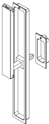
Manilla plana interior con uñero exterior Ref.: H13045
