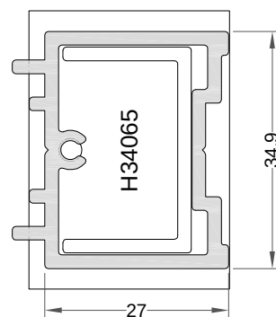
Unión 4 hojas Ref.: 7910
