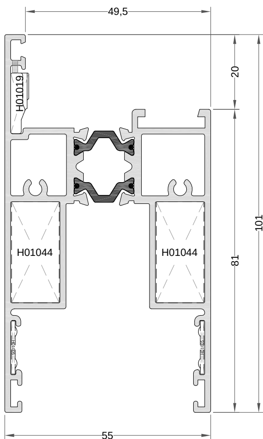
Hoja perimetral Ref.: 7904
