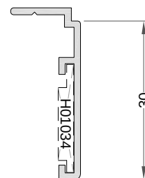
Solape compacto 30 Ref: 7130
