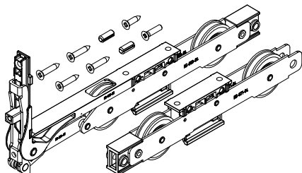
Kit carros Elevable (300 Kg/Hoja) Ref.: H32035
