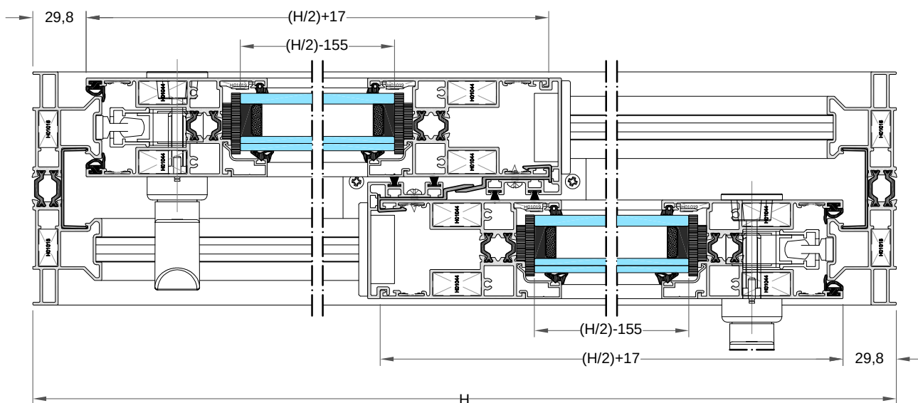
Sección horizontal
