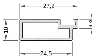
Reductor hoja minimalista Ref.: 7916
