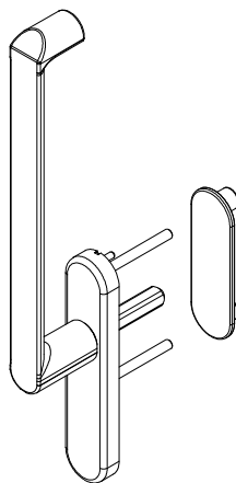
Manilla interior sin bocallave y roseta exterior Ref.: H13042
