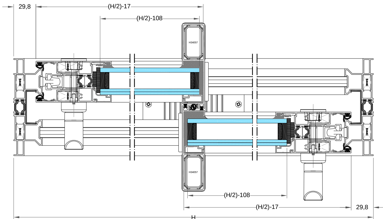
Sección horizontal
