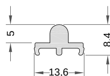
Carril de rodadura Ref.: 7902
