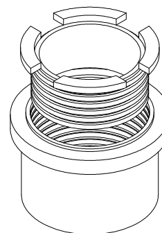
Embudo bajante Ref.: H35008
