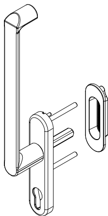
Manilla interior con bocallave y uñero exterior Ref.: H13041
