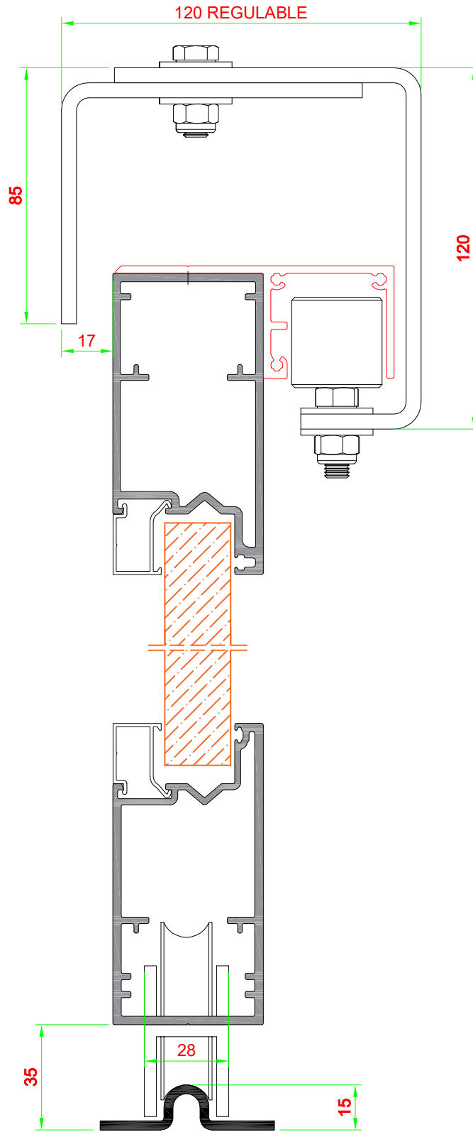
SECCION VERTICAL
