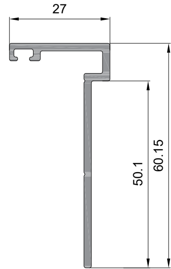
Perfil Batiente Ref:1646
