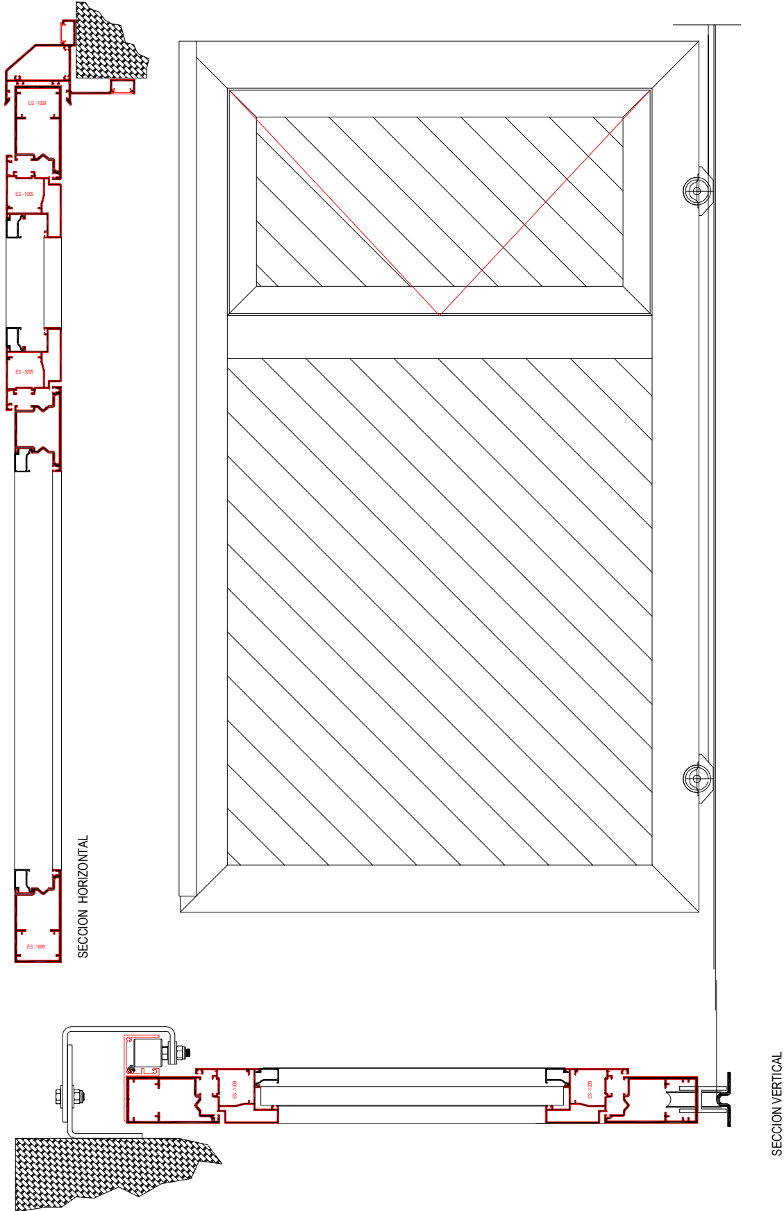
Secciones Puerta corredera con postigo
