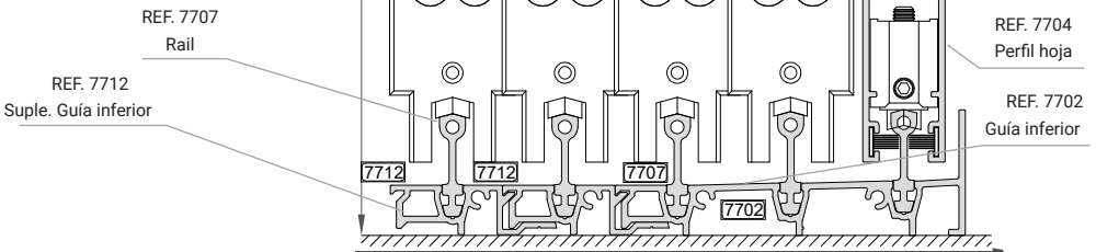
SECCIÓN VERTICAL
