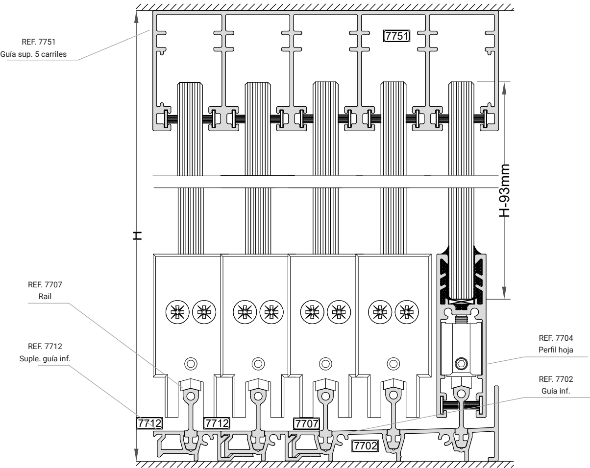
SECCIÓN VERTICAL
