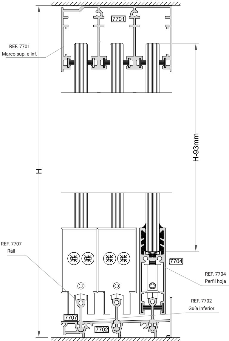
SECCIÓN VERTICAL
