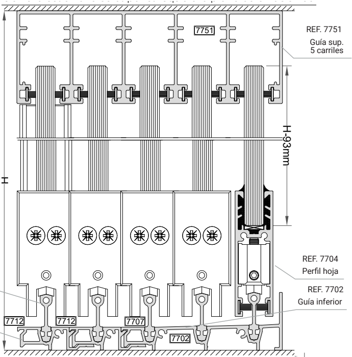
SECCIÓN VERTICAL
