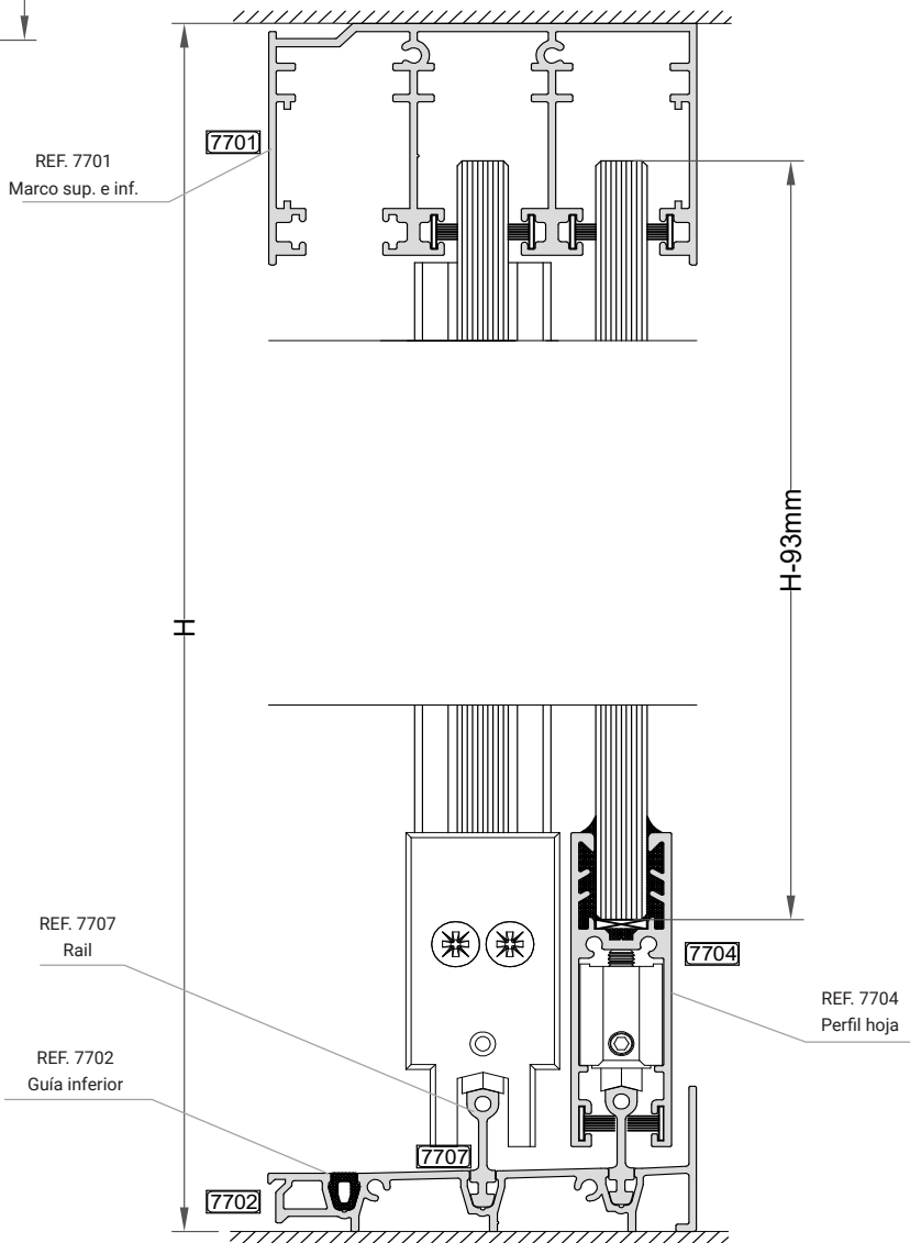
SECCIÓN VERTICAL
