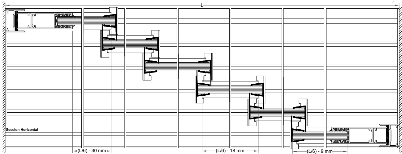
SECCIÓN HORIZONTAL
