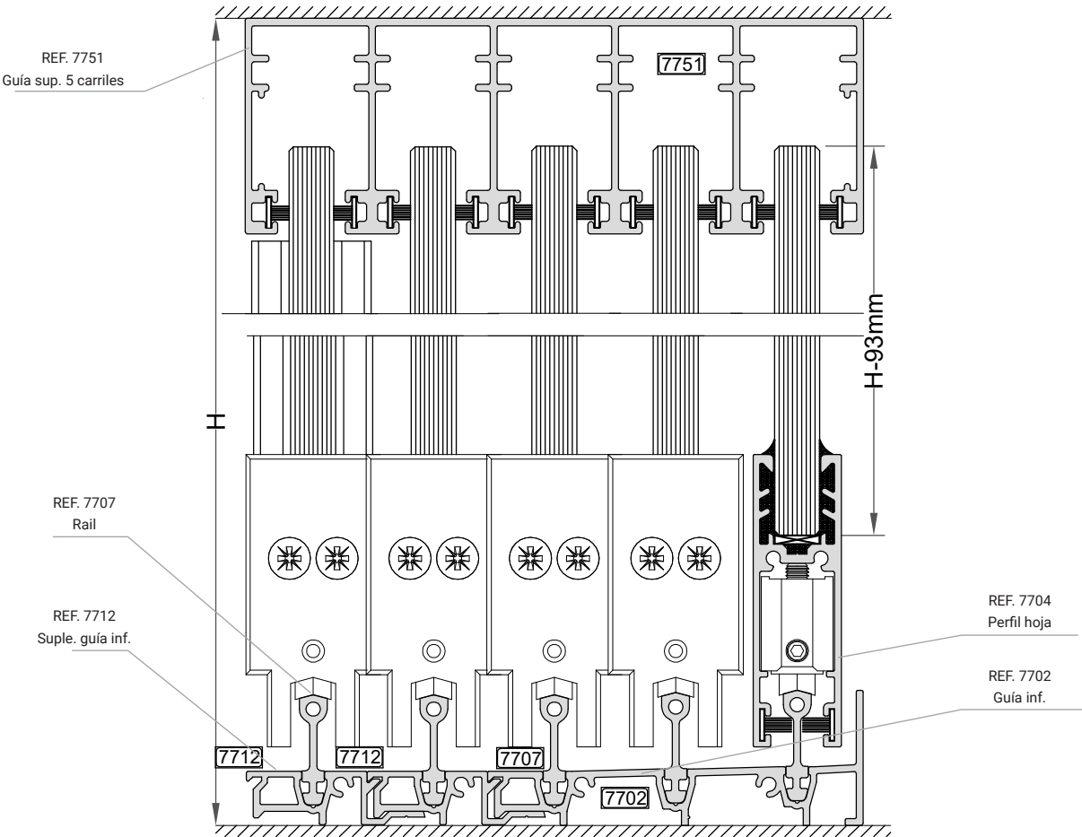
SECCIÓN VERTICAL
