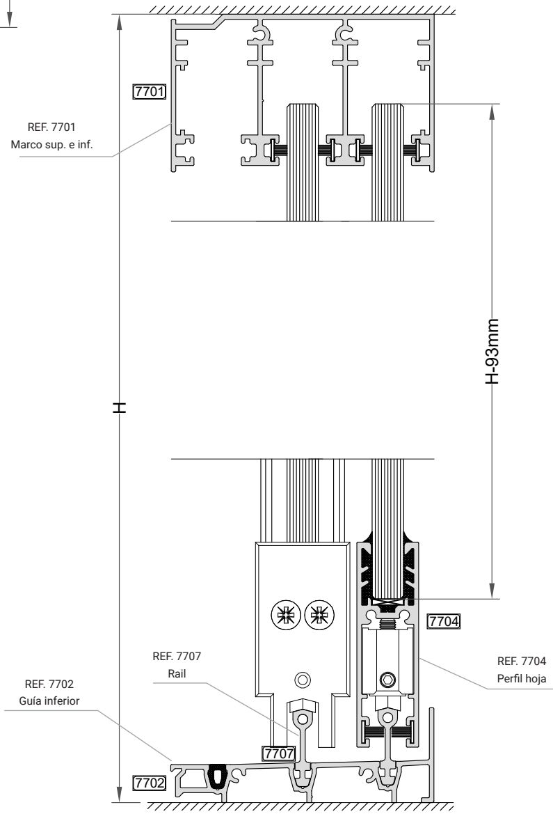
SECCIÓN VERTICAL
