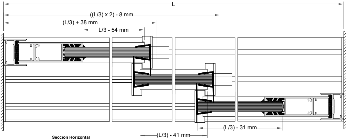
Seccion Horizontal
