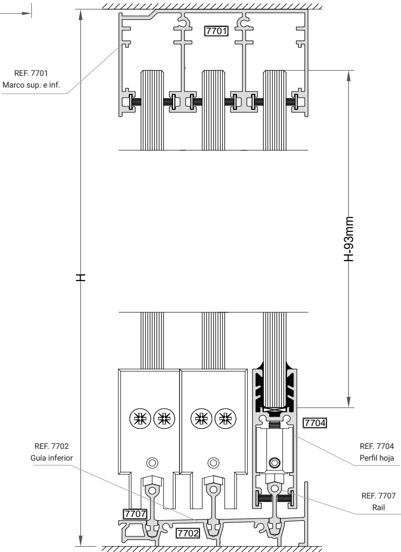
SECCIÓN VERTICAL
