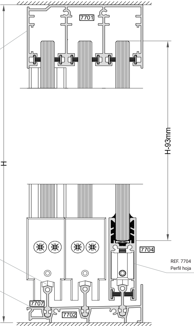
SECCIÓN VERTICAL
