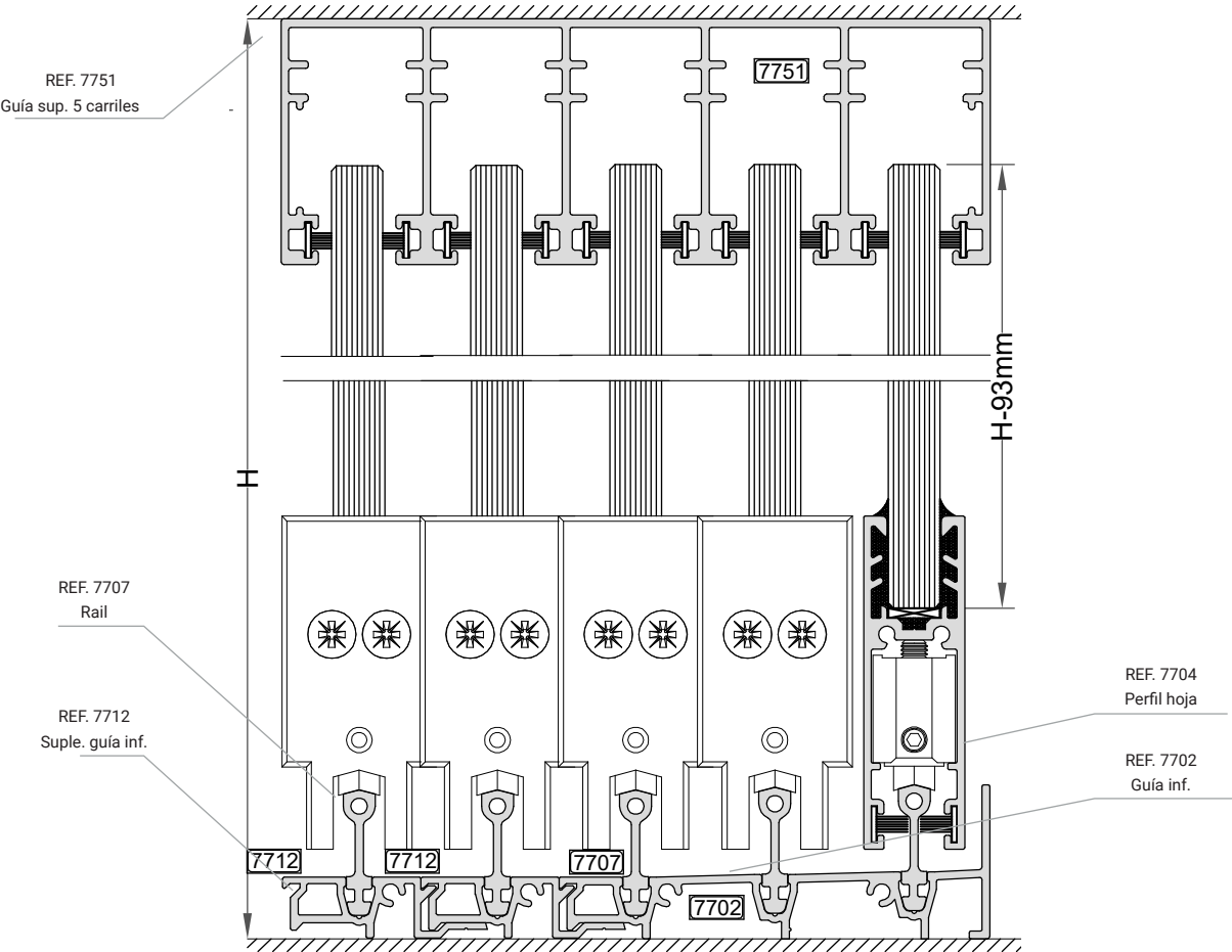
SECCIÓN VERTICAL
