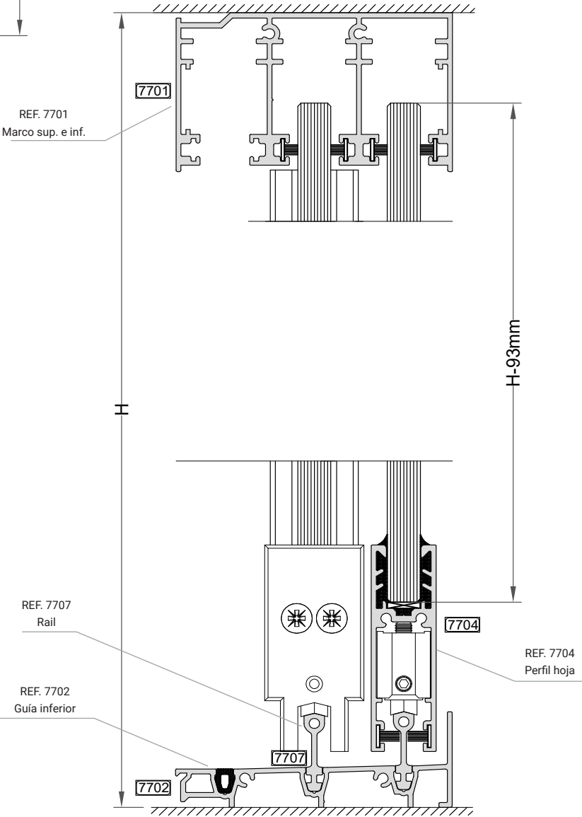
SECCIÓN VERTICAL
