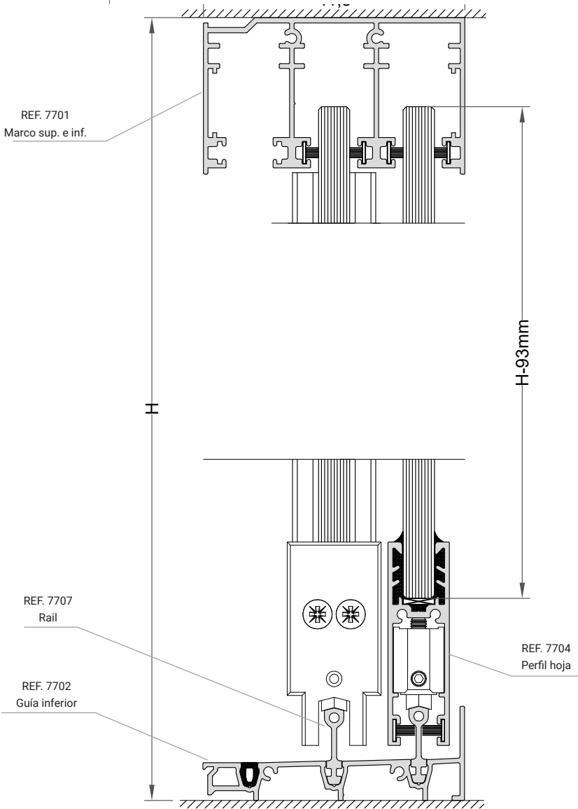
SECCIÓN VERTICAL
