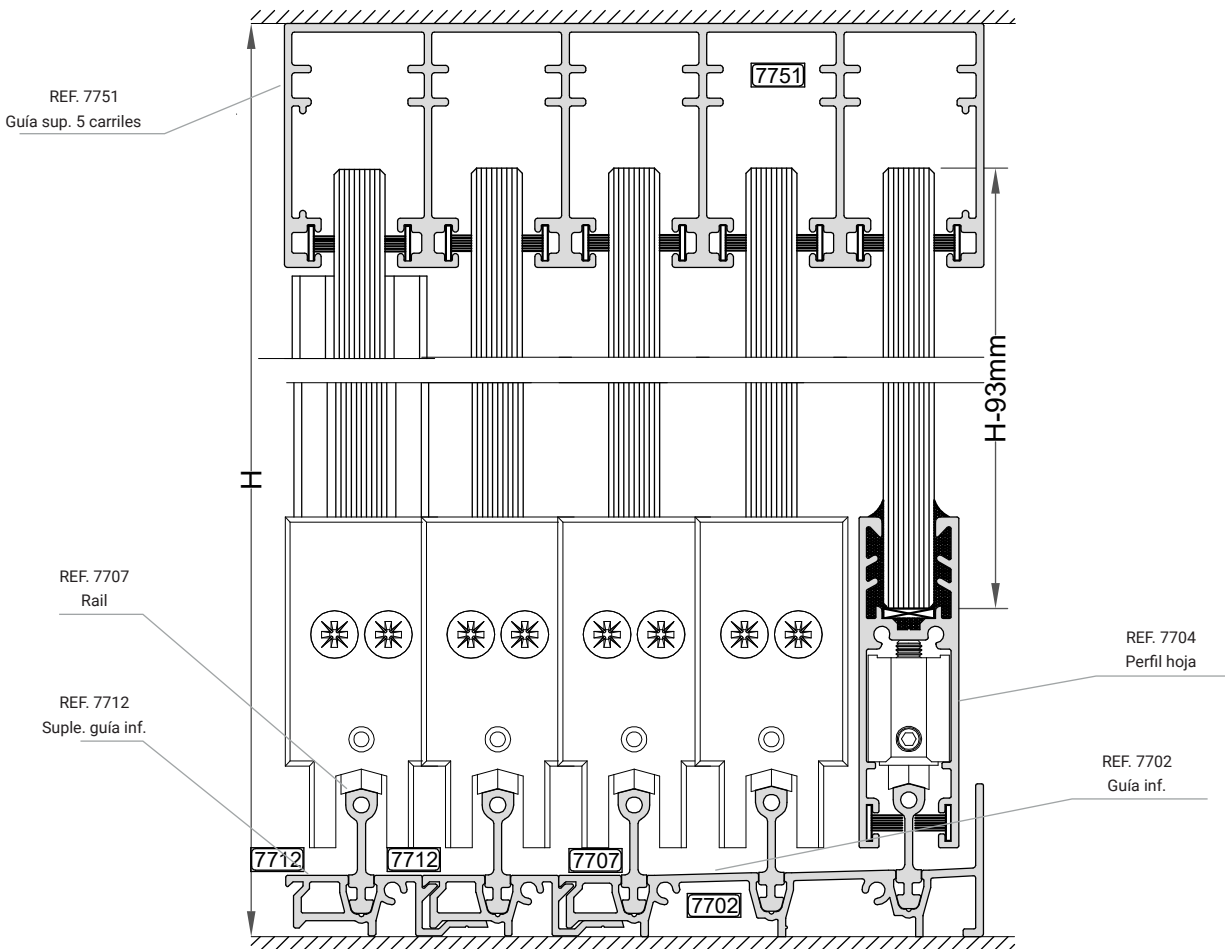
SECCIÓN VERTICAL
