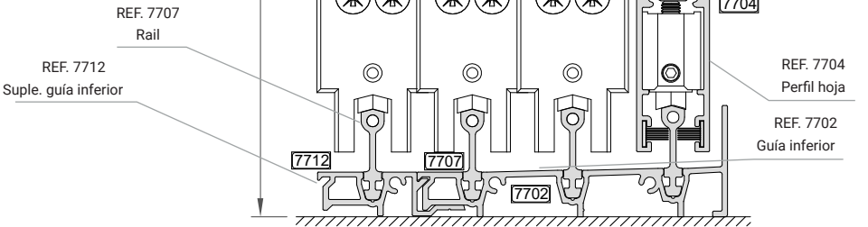
SECCIÓN VERTICAL
