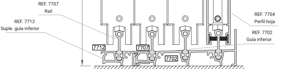
SECCIÓN VERTICAL
