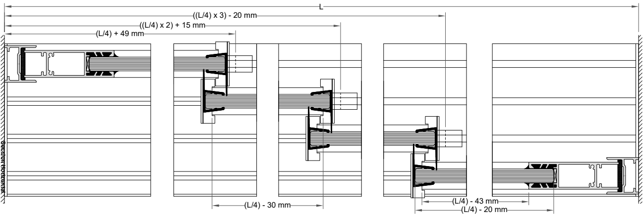
SECCIÓN HORIZONTAL
