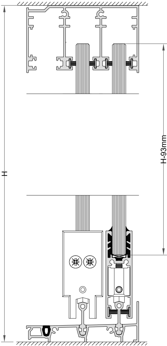
SECCIÓN VERTICAL
