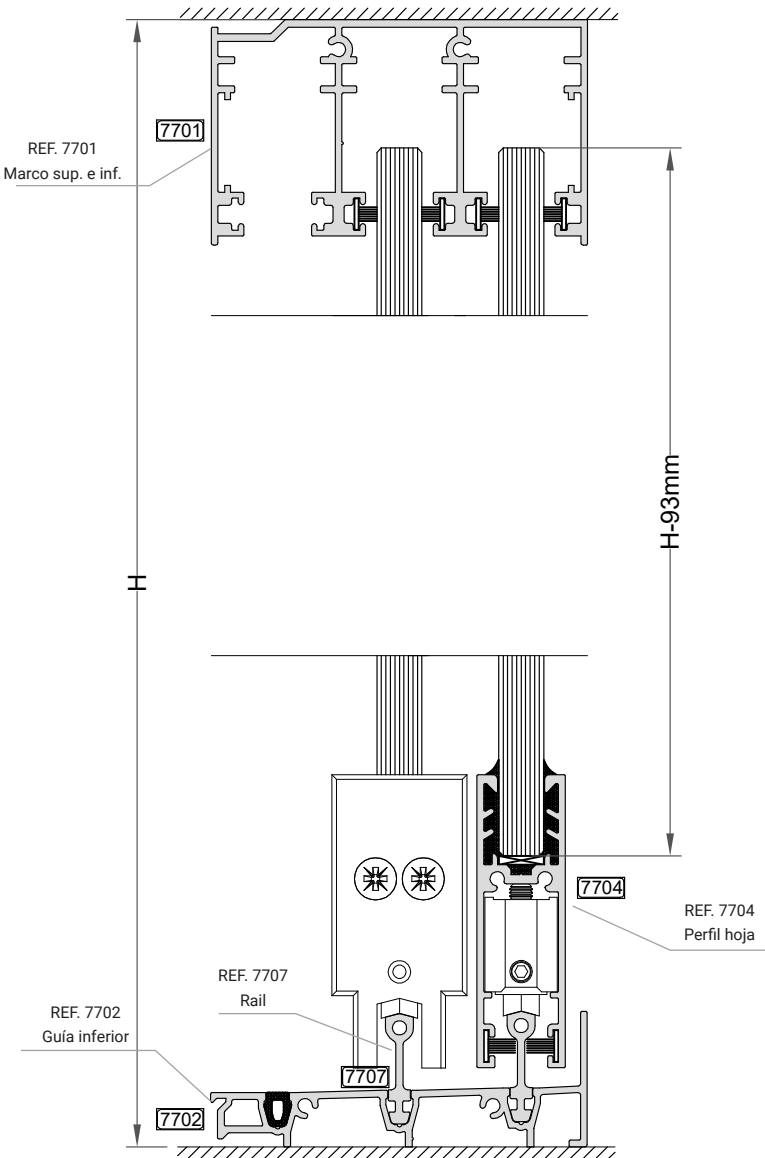
SECCIÓN VERTICAL
