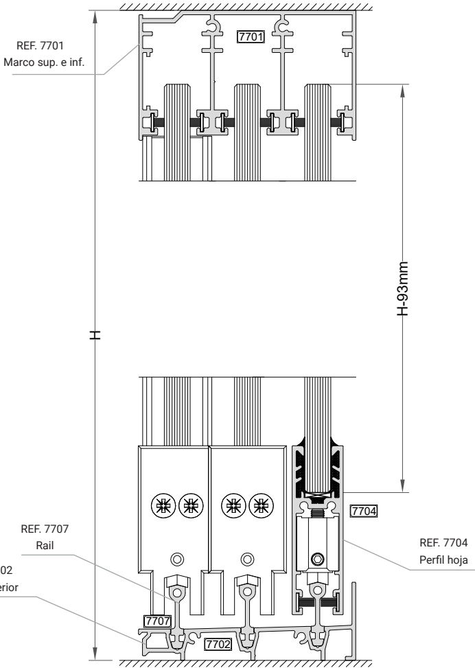
SECCIÓN VERTICAL
