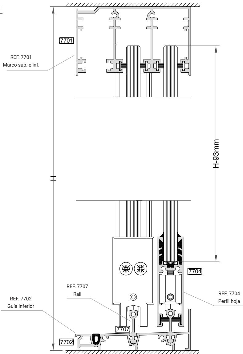
SECCIÓN VERTICAL
