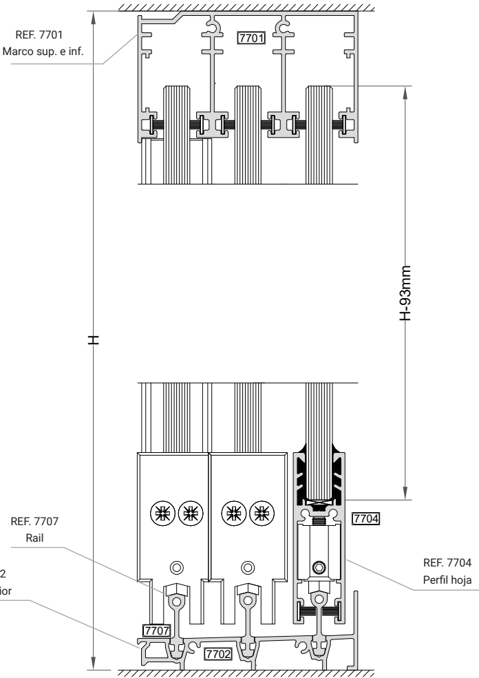
SECCIÓN VERTICAL
