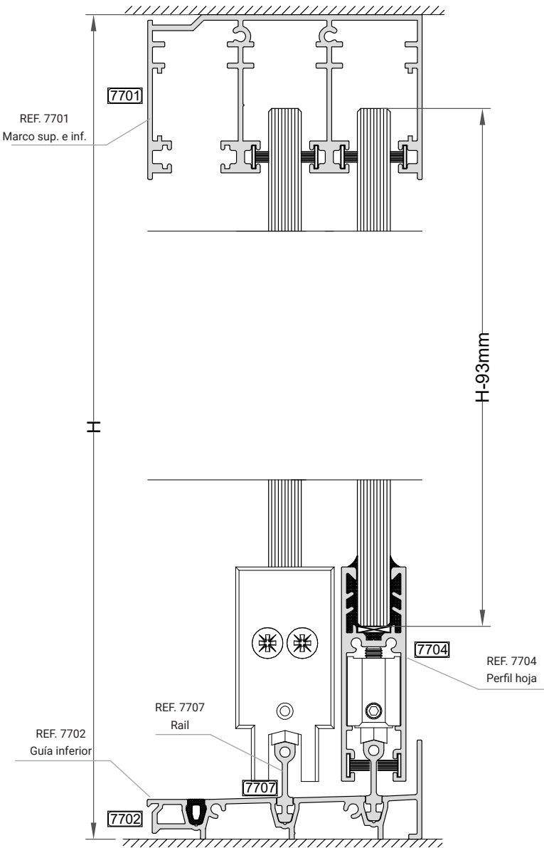
SECCIÓN VERTICAL
