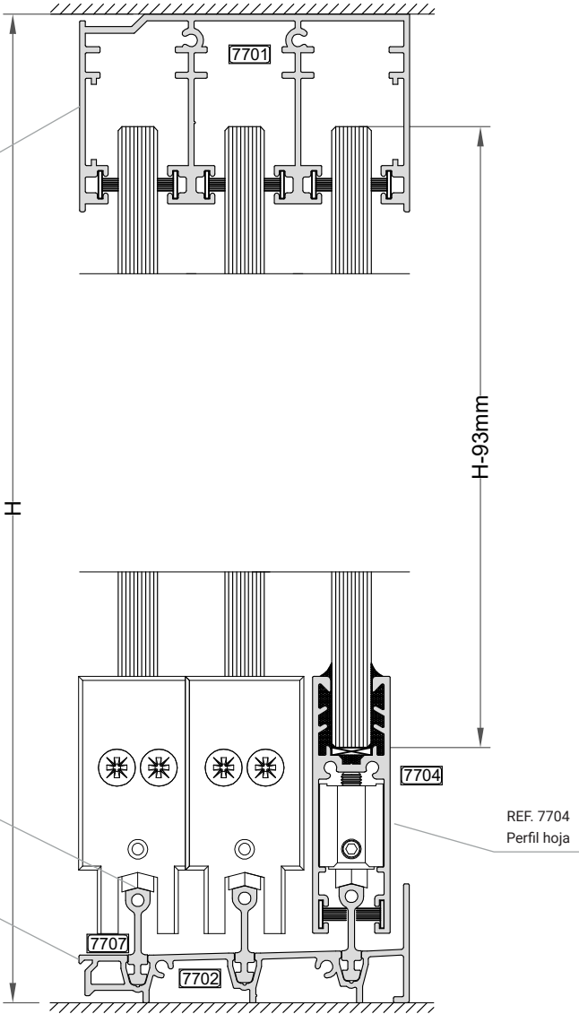
SECCIÓN VERTICAL
