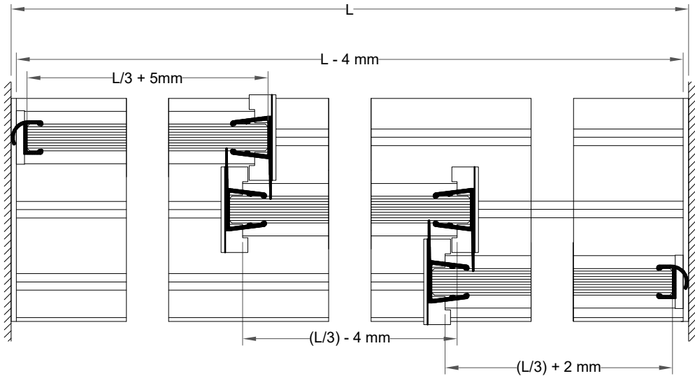
SECCIÓN VERTICAL
